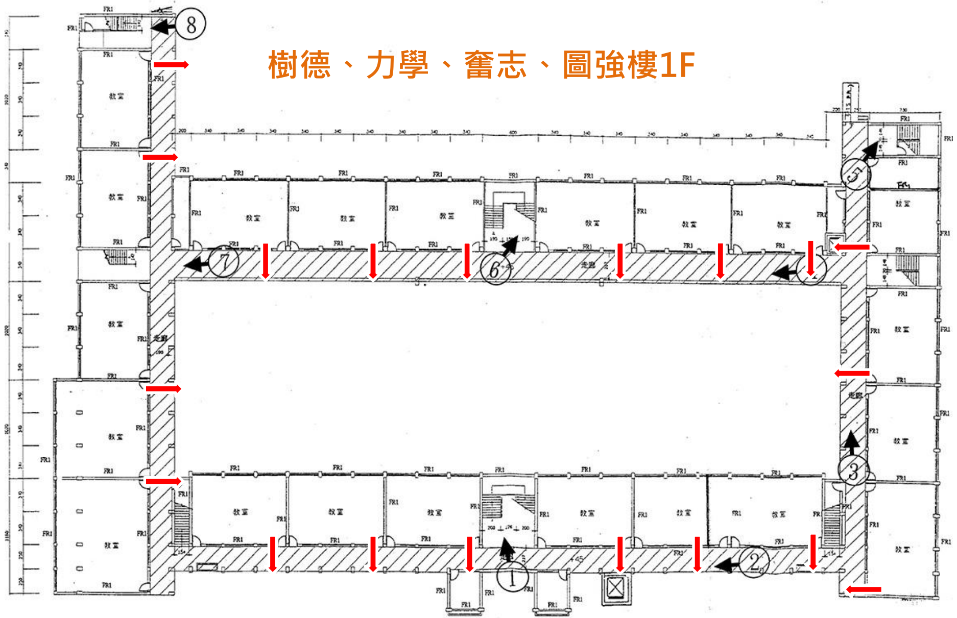
②③棟一樓平面圖
