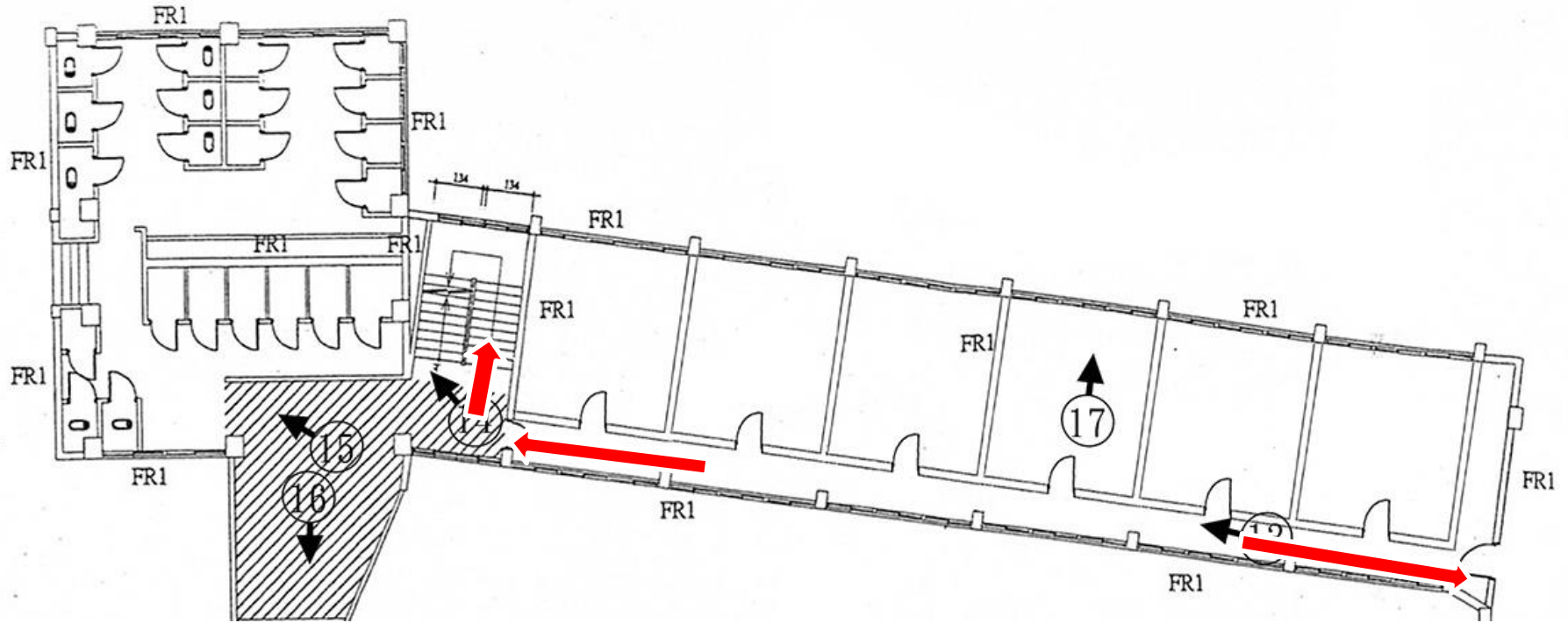
三樓平面圖
