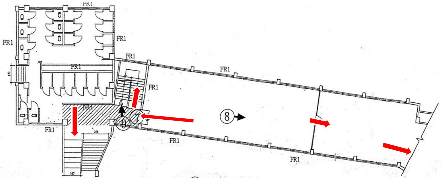
⑧棟二層平面圖
