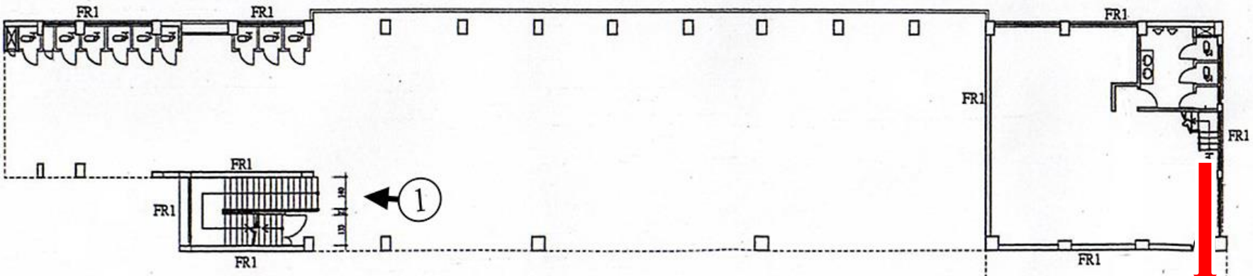
④ 棟一層平面圖
