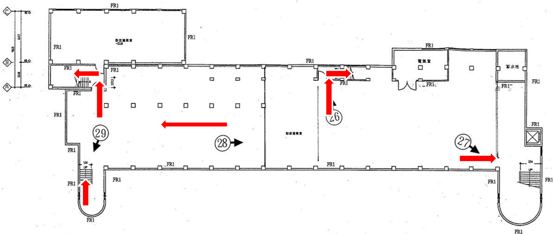
9 10 棟地下室平面圖
